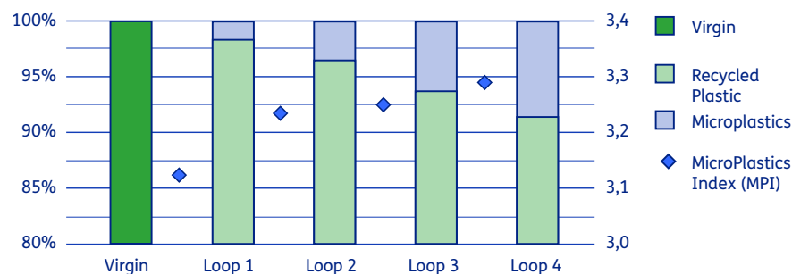
Figuur 7. MicroPlastics Index ♦ en massabalans (kolom) van multiple-loop experiment TNO met polypropyleen. Bron: TNO.
